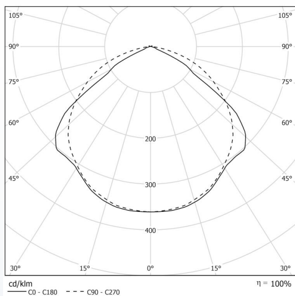
Křivka svítivosti svítidla ALPHA ES INDUSTRY SLIM CL asymetrické vyzařování při 4 000K
