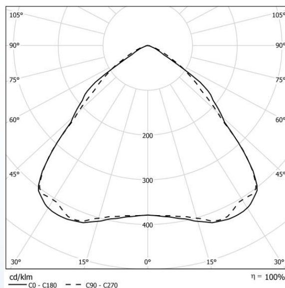
Křivka svítivosti svítidla ALPHA ES INDUSTRY SLIM CLM asymetrické vyzařování při 4 000 K, umístěna mřížka proti oslnění
