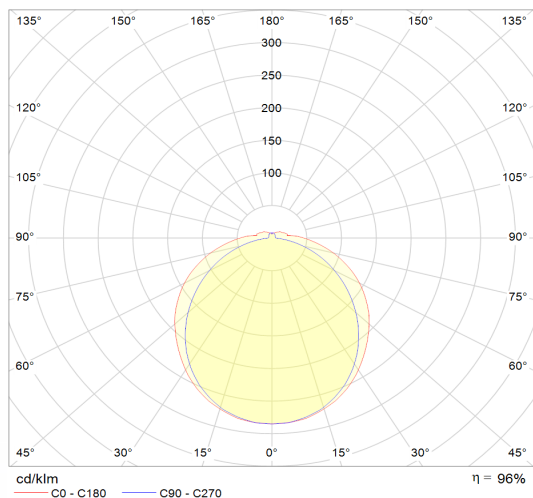
Křivka svítivosti
